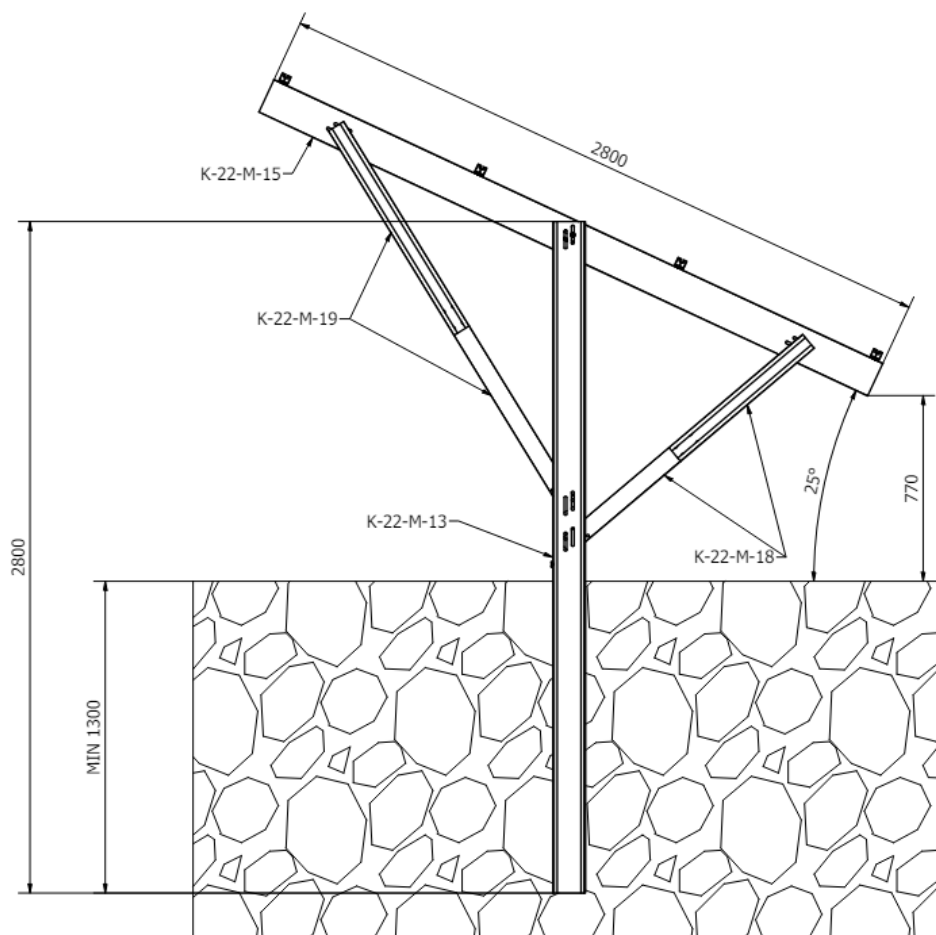
Rys.1 Wymiary konstrukcji
